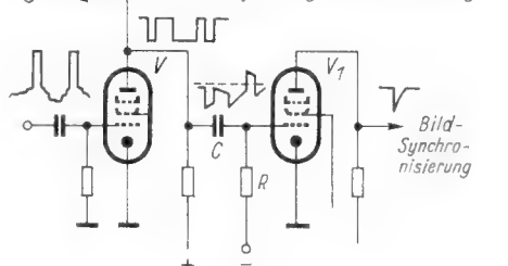
Unten: Bild 159. Prinzipschaltung für die Rückfrontsynchronisierung
