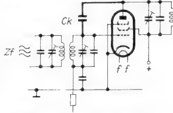
Mit einem Drahtkondensator Ck entdämpfte Zf-Stufe
