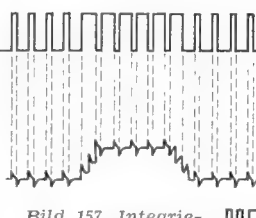
Bild 157. Integrierende Wirkung des Tiefpasses nach Bild 155
