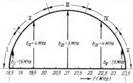
Bild 56. Zeichnerische Ermittlung der Abgleichfrequenzen für einen mehrkreisigen Zf-Verstärker
