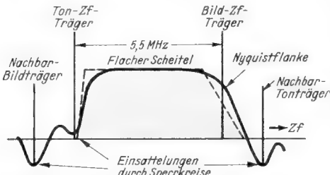
Bild 54. Theoretische Zf-Durchlaufkurve (gestrichelt) und praktisch erzielte Annäherung (ausgezogen)
