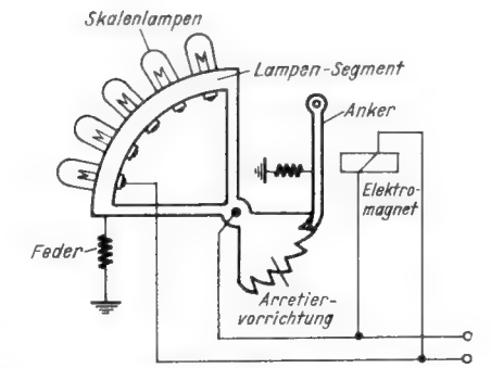
Ausführungsbispiel des Automaten zum Einschalten von Reserve-Skalenlampen
