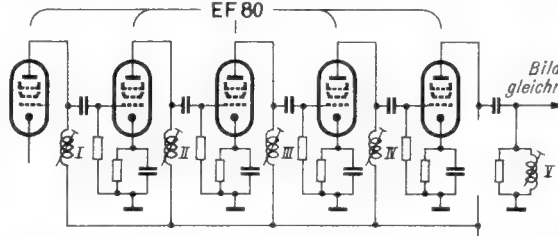
Bild 55. Vierstufiger gestaffelt abgestimmter Zf-Verstärker
